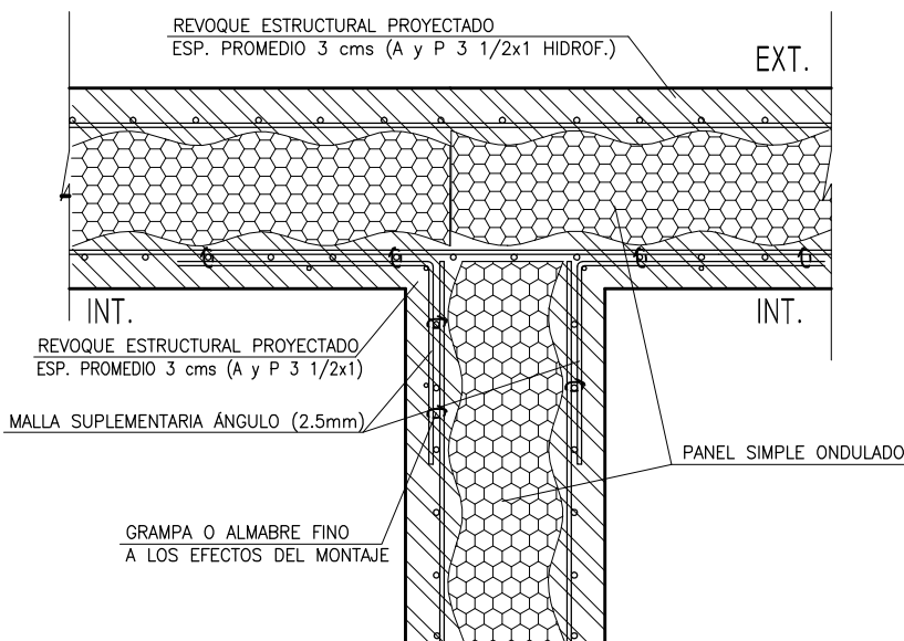
D3 ENCUENTRO DE DOS PANELES EN "T"
