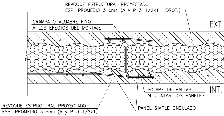
D1 ENCUENTRO DE DOS PANELES CONTIGUOS
