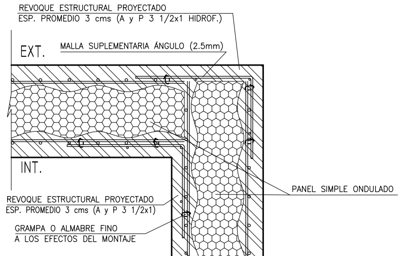
D2 ENCUENTRO DE DOS PANELES EN "L"
